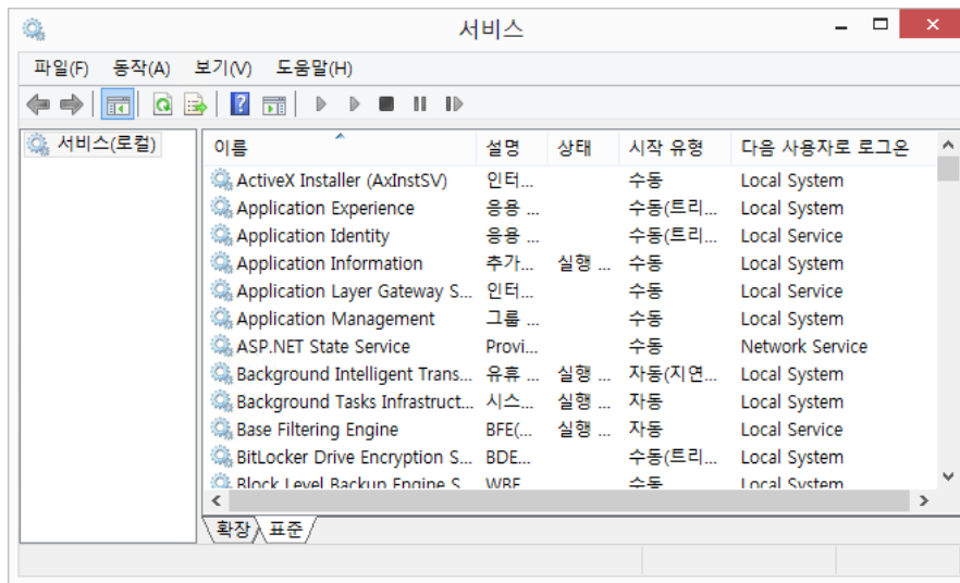
그림 14.53 서비스 목록
