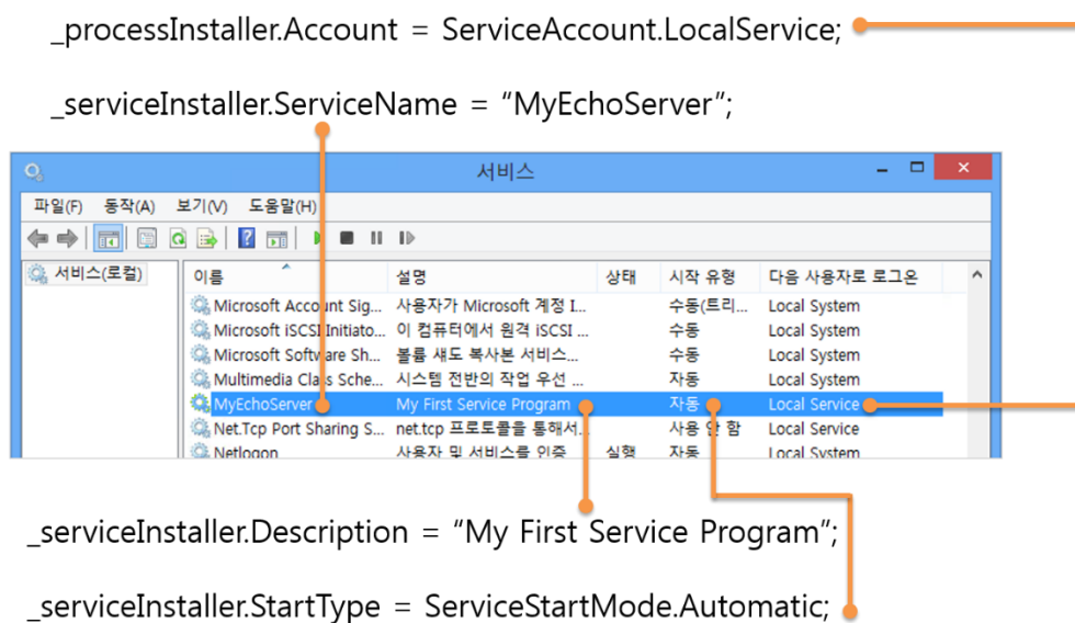
그림 18.54 서비스 관리자에 설정되는 변수의 값
