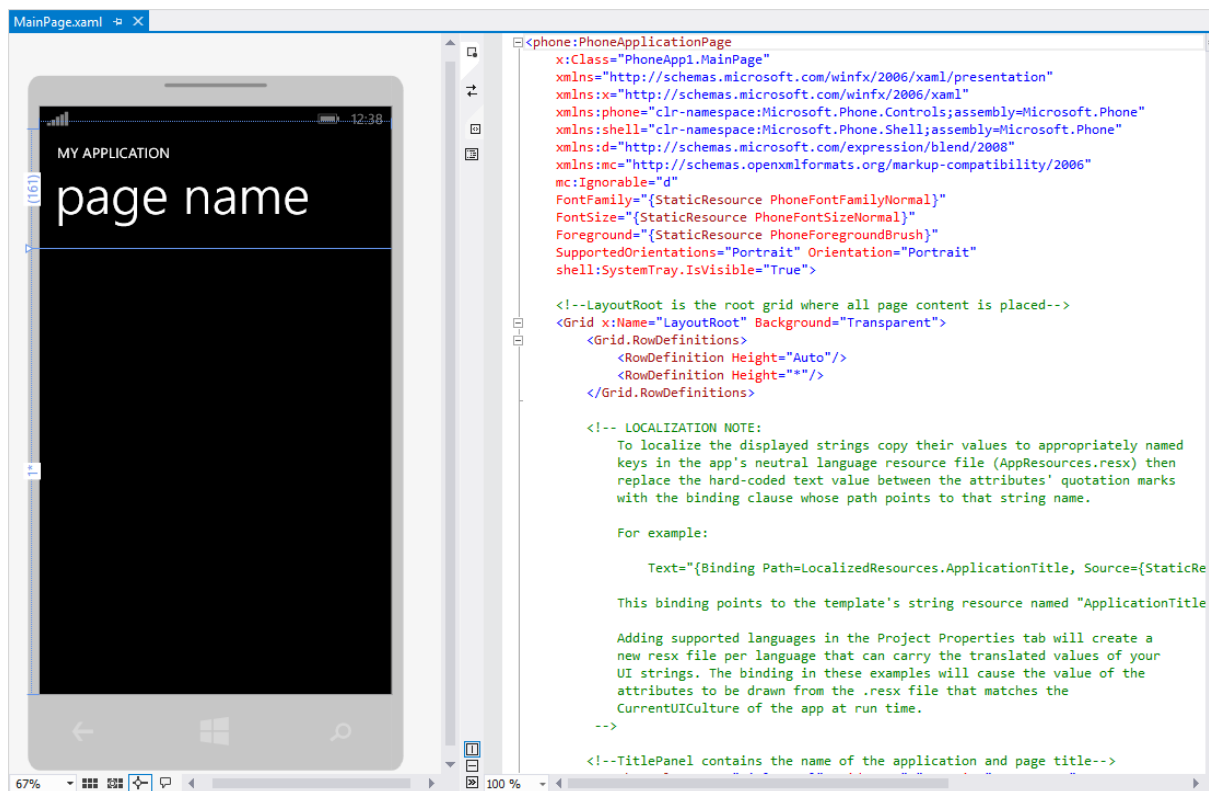
그림 18.77 MainPage.xaml 편집 및 디자인 화면
