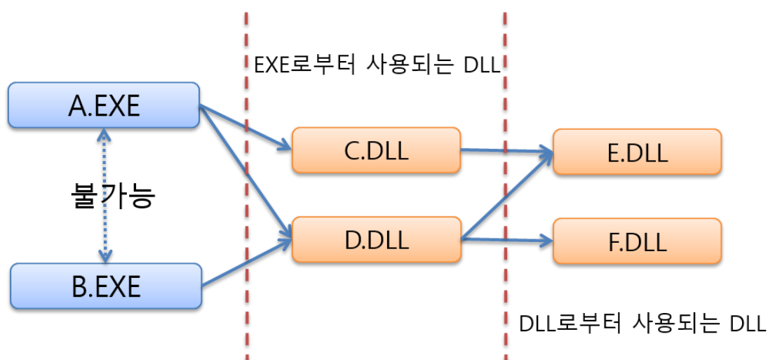
그림 E.6 DLL과 EXE의 참조 관계
