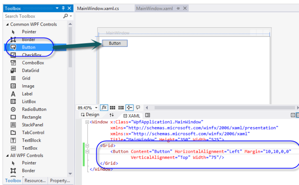
그림 18.39 Button 컨트롤을 추가
