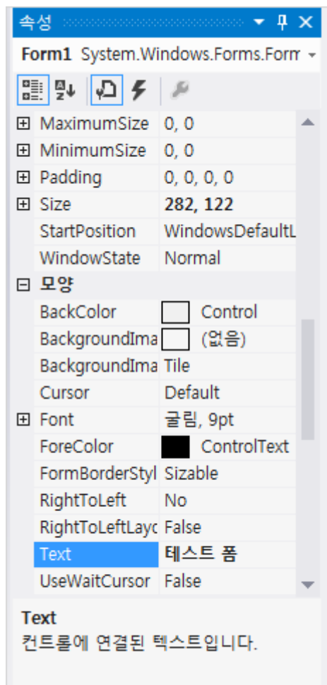
그림 18.7 디자인 창에 선택된 객체의 속성을 보여주는 속성창
