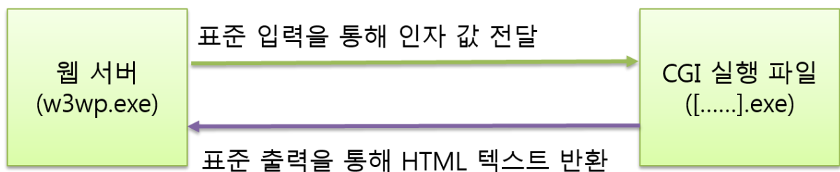
그림 18.57 CGI 동작 방식
