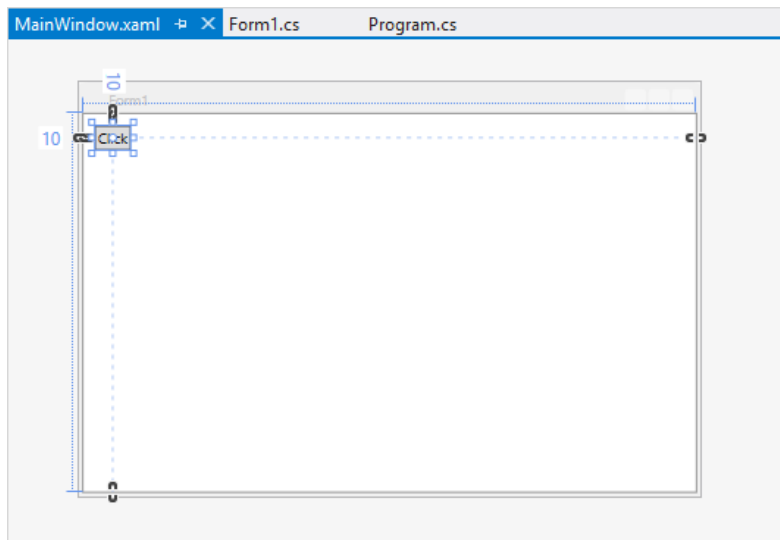
그림 18.47 Margin="10, 10, 0, 0"을 지정한 컨트롤 위치
