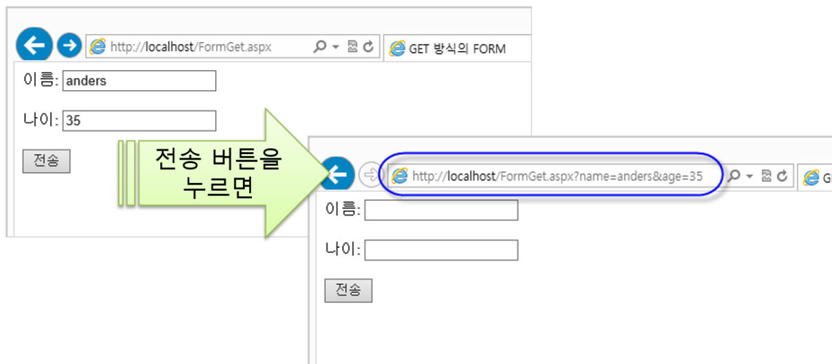
그림 18.61 GET 방식을 이용한 FORM 데이터 전송
