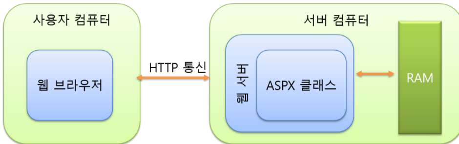
그림 18.65 웹 응용 프로그램의 실행 구조
