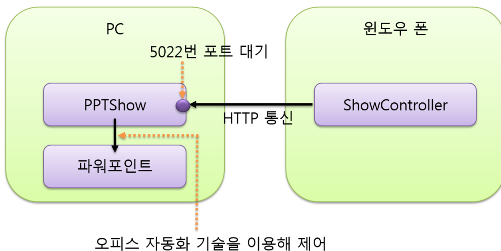
그림 19.2 세부 동작 구조
