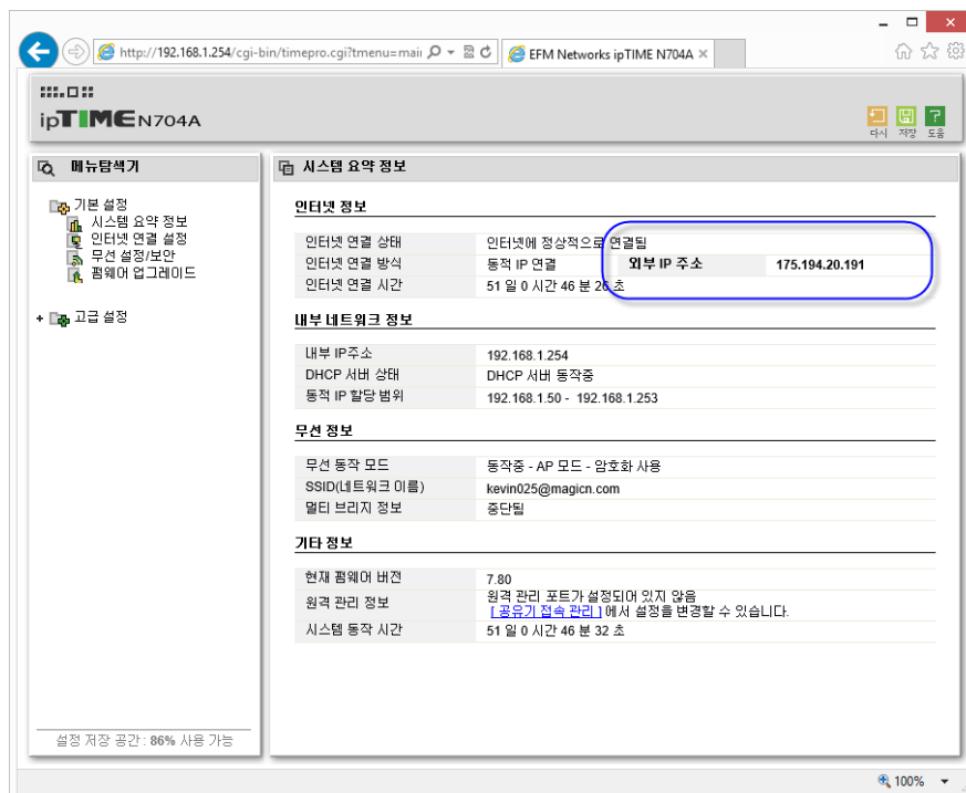
그림 18.73 공유기의 관리자 홈페이지를 이용한 공용 IP 주소 확인
