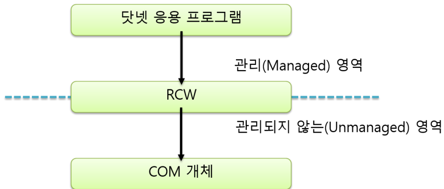
그림 19.12 RCW의 구조
