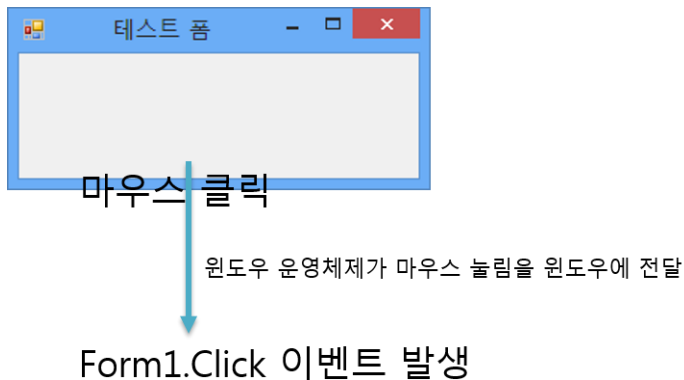
그림 18.8 윈도우 폼 이벤트 발생
