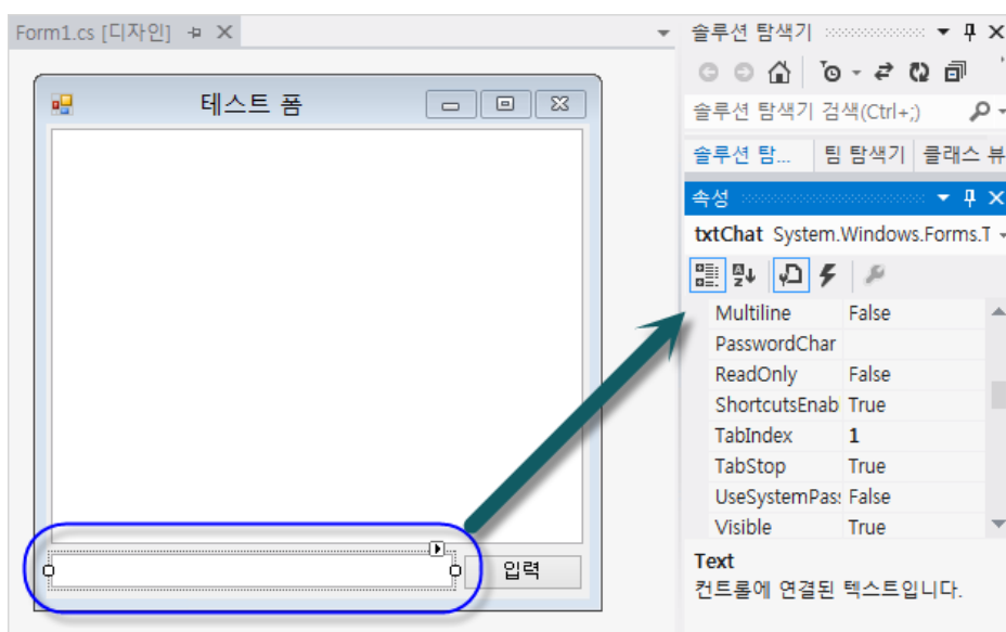
그림 18.12 선택된 컨트롤의 속성 창 정보
