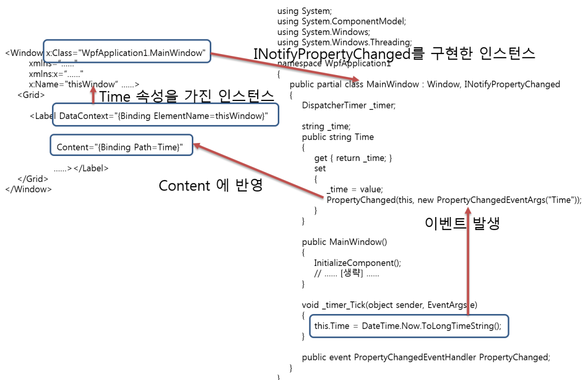
그림 18.42 WPF 데이터 바인딩
