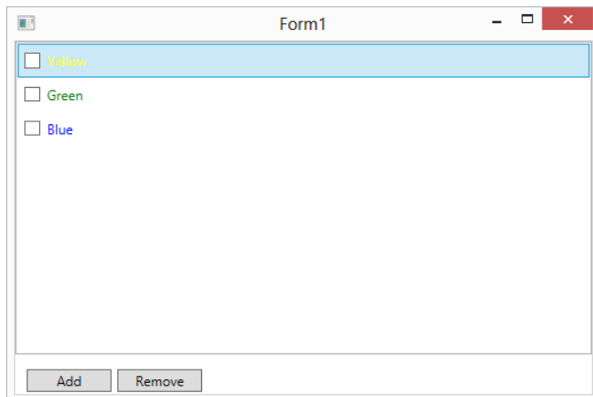
그림 18.52 Foreground 속성에 바인딩된 글자 색
