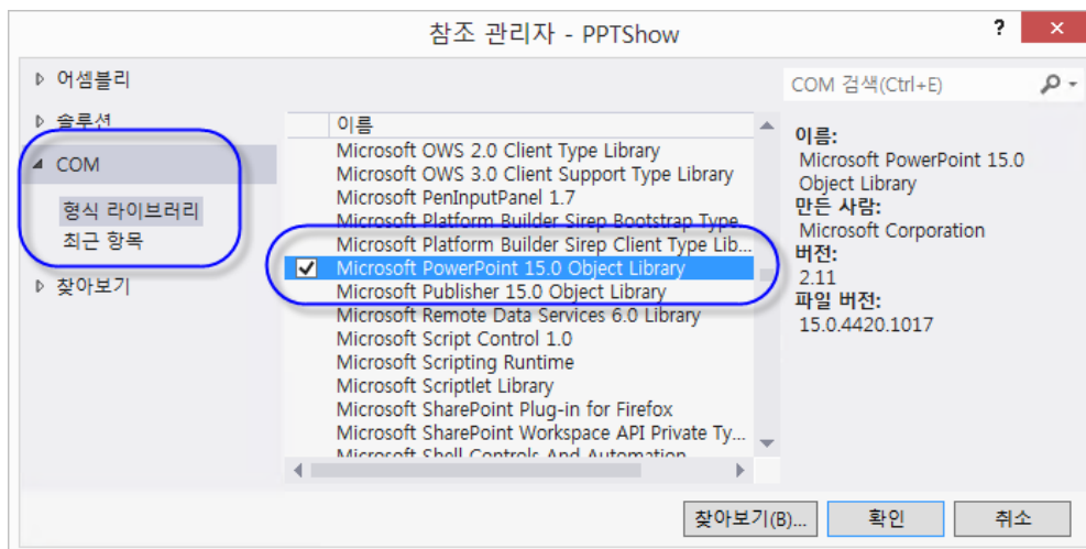
그림 19.13 파워포인트 COM 개체의 RCW 생성을 위한 참조 추가
