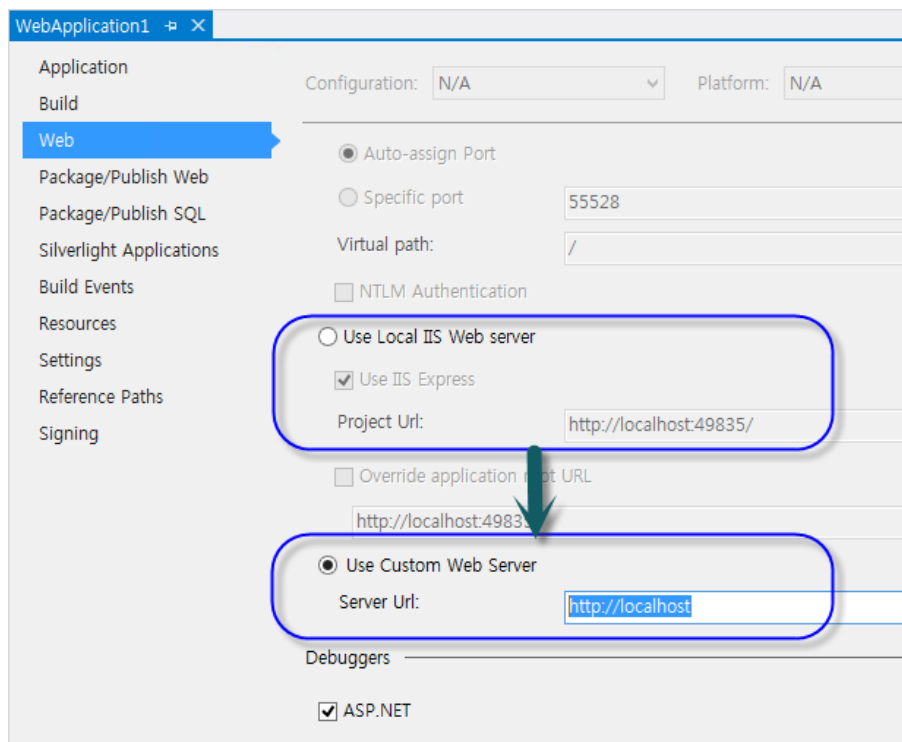
그림 18.71 IISExpress에서 IIS로 호스팅 환경을 전환
