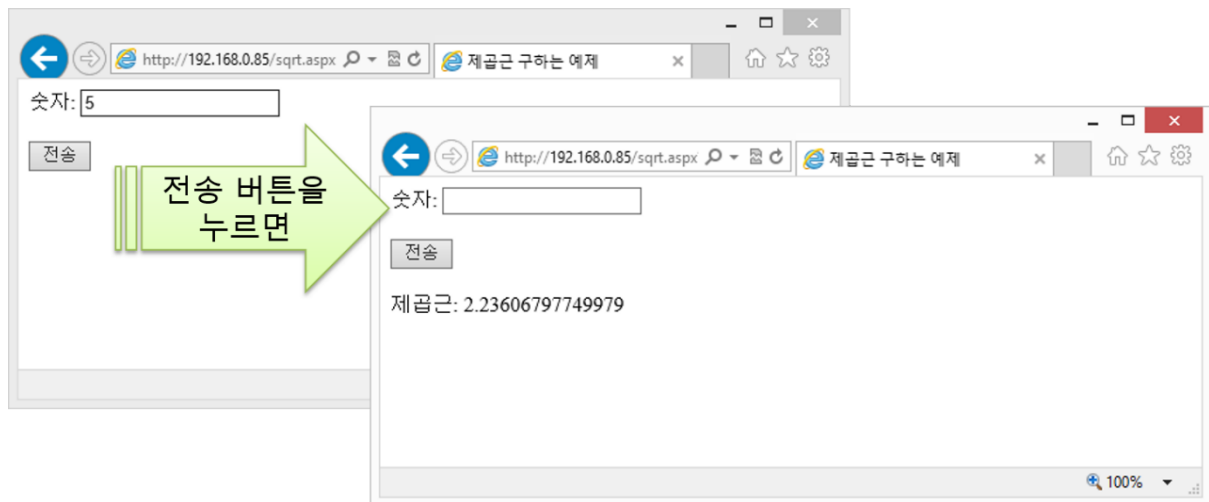
그림 18.66 폼을 submit 한 경우
