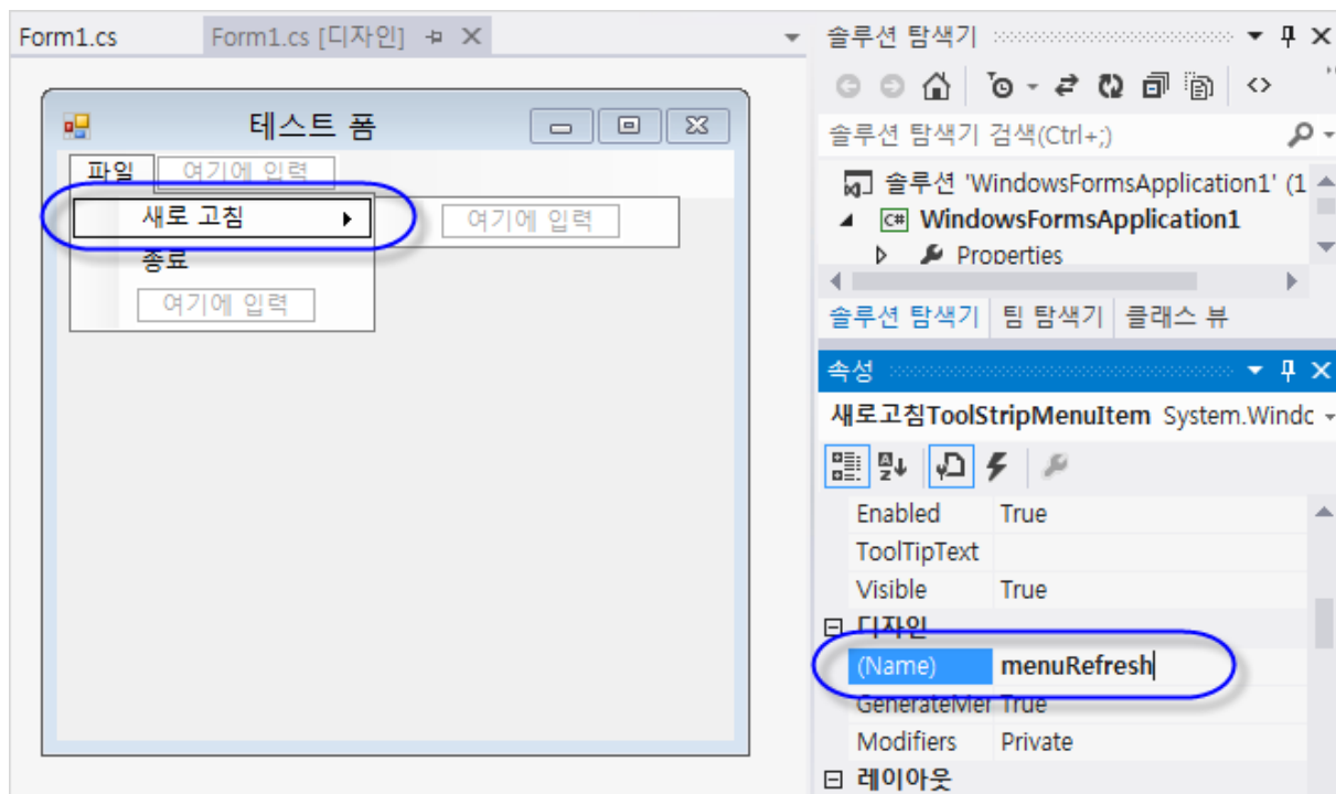
그림 18.18 "새로 고침" 메뉴의 (Name) 항목 편집
