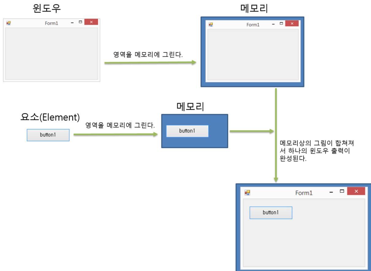
그림 18.41 WPF의 출력 구성
