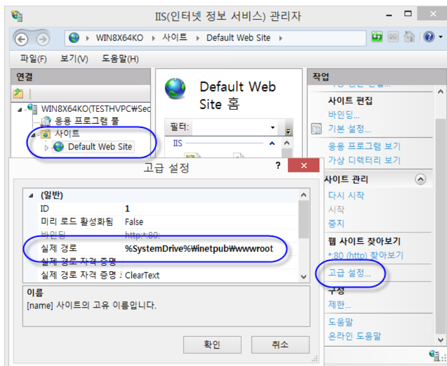
그림 18.56 IIS 관리자에서 사이트 고급 설정을 통해 경로를 확인
